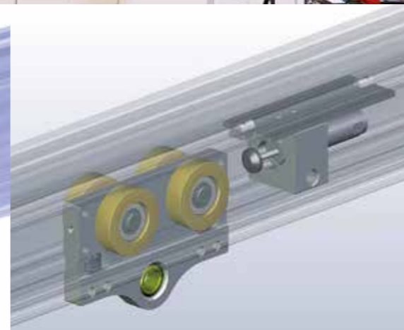
Carrello del paranco e respingente idraulico regolabile
